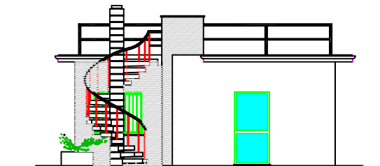
Prospetto Ovest
