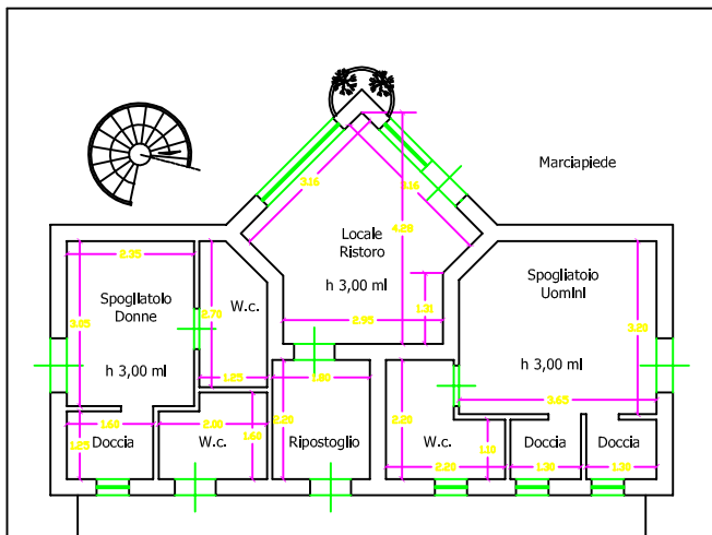
Pianta Terra
